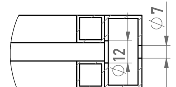
DETAIL B M: 1 : 2
